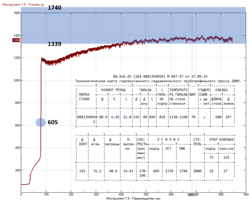
Рис. 12 – Графік розподілу сили пресування, залежно від переміщення голки для труби. 88,9 x 6, 45 мм
