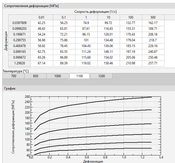
Рис. 7 – Характеристики марок сталей: а – 12X18Н10Т, б – 12X13
