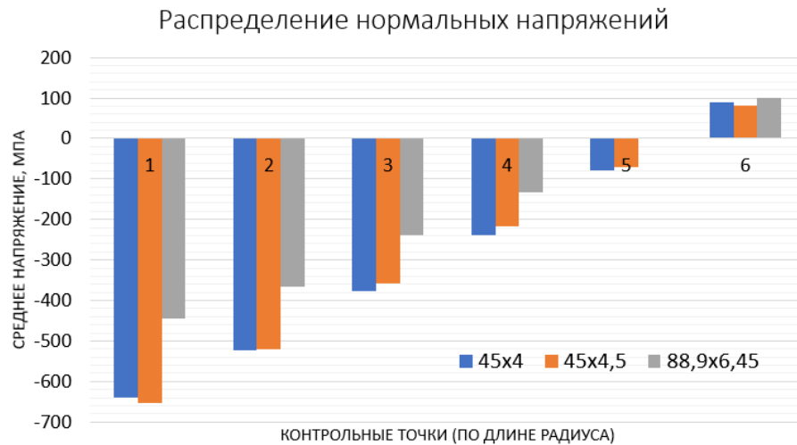
Рис. 21 - Графік розподілу нормальних напруг
