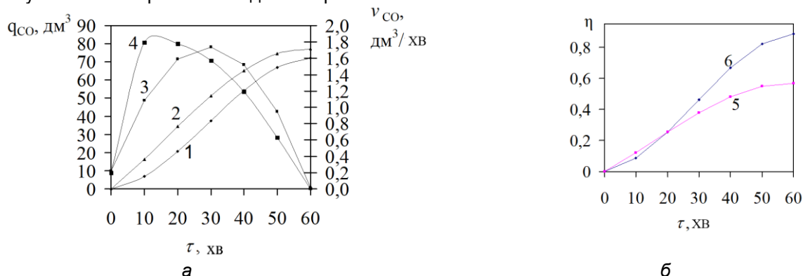
Рис. 2. Термокінетичні криві доновлення SiO 2 з вторинних матеріалів вуглецем: а – 1 і 2 – сумарна кількість CO, що виділився (відвальна шихта виробництва абразивного карбіду кремнію + графіт (1) і вуглецькарбідокремнієва суміш електродного виробництва + відвальна шихта виробництва абразивного карбіду кремнію; 3 та 4 – швидкість виділення CO при відновленні шихти №1 та №2 відповідно; б – 5 та 6 – ступінь відновлення шихти №1 та №2 відповідно
