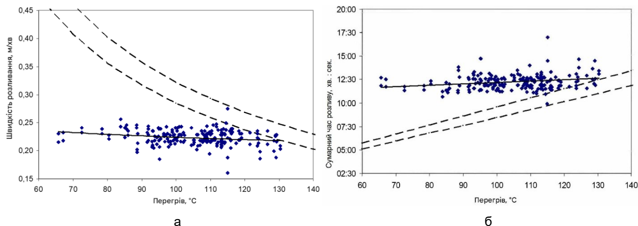
Рисунок 2 – Зміна швидкості (а) і часу (б) розливу злитків залежно від перегріву сталі над температурою лідідус: — фактична крива - - - розрахунковий інтервал
