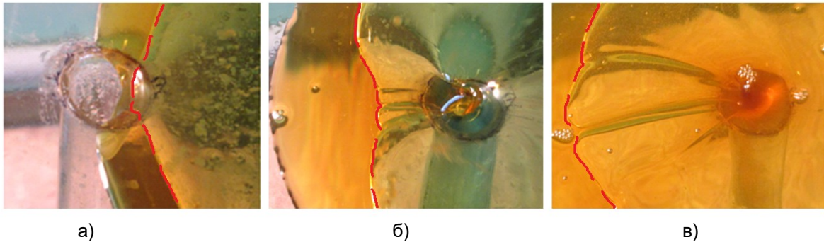
Рисунок 3. Кінограма нахилу конвертера до випуску і відповідно виливу рідкої ванни через сталевипускний канал льотки конвертера (фізичне моделювання – вільний вилив): а) 1 сек. виливу, б) 20 сек. виливу, в) 25 сек. виливу; червоний контур – межа розділу фаз шлак/метал.
