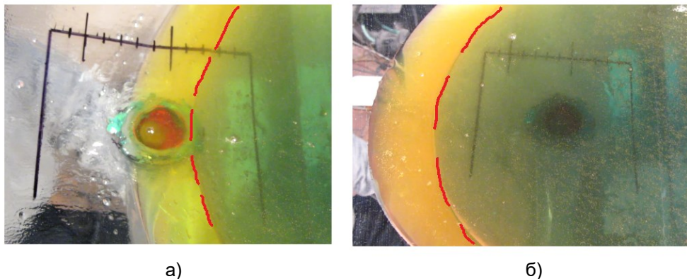
Рисунок 4. Кінограма нахилу конвертера до випуску і відповідна затримка виливу рідкої ванни через сталевипускний канал льотки (фізичне моделювання – пластичний стопор первинного відсікання): а) 1 сек. виливу, б) 5 сек. виливу; червоний контур – межа розділу фаз шлак/метал.
