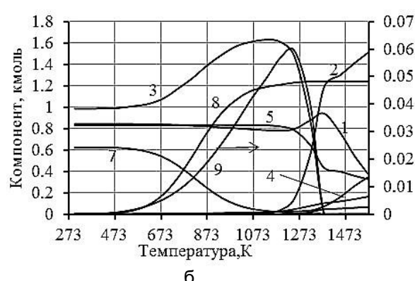
Рис. 3. Термодинамічне моделювання процесу газифікації \text{Cr}_3\text{C}_2 комплексним окислювачем а) ( \text{H}_2\text{O} + \text{CO}_2 ) і б) ( \text{H}_2\text{O} + \text{CO}_2 + \text{O}_2 ): 1 – \text{Cr}_3\text{C}_2 ; 2 – \text{CO} ; 3 – \text{C} ; 4 – \text{Cr}_7\text{C}_3 ; 5 – \text{Cr}_2\text{O}_3 ; 6 – \text{Cr}_{23}\text{C}_6 ; 7 – \text{CH}_4 ; 8 – \text{H}_2 ; 9 – \text{Cr}
