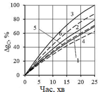
Рис. 5. Вплив газоподового складу на кінетику газифікації різних вуглецевих матеріалів при 1273K: 1, 2, 3 – деревне вугілля; 4, 5, 6 – піролігнін; 1, 4 – 70% \text{CO}_2 + \text{Ar} ; 2, 5 – 70% \text{CO}_2 + \text{H}_2 ; 3, 6 – 70% \text{CO}_2 + \text{H}_2\text{O}
