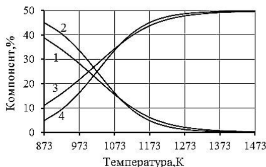
Рис. 2. Рівноважний склад газової фази газифікації \text{Cr}_3\text{C}_2 водяною парою і \text{CO}_2 для реакції 5 і 6: 1 – \text{H}_2\text{O} , 2 – \text{CO}_2 , 3 – \text{H}_2 і 4 – \text{CO}
