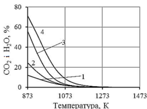
Рис. 1. Рівноважний склад газової фази вуглецевої газифікації становить 1,2 – \text{H}_2\text{O} , 3,4 – \text{CO}_2 при: 1 – \alpha=0,75 і \beta=0,25 ; 2 – \alpha=0,25 і \beta=0,75 ; 3 – \alpha=0,25 ; 4 – \alpha=0,75 при цьому \alpha = (P_{\text{CO}_2} + P_{\text{CO}}) ; \beta = (P_{\text{H}_2} + P_{\text{H}_2\text{O}})
