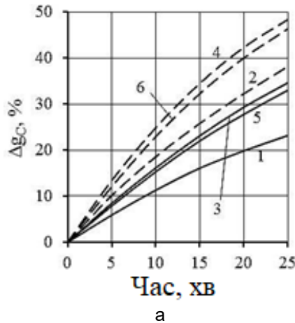
Рис. 6. Вплив добавок на кінетику газифікації графіту (а) і піролігніну при 1273 К різними газами: 1, 3, 5 – CO 2 ; 2, 4, 6 – H 2 O; 1, 2 – без добавок; 3, 4 – 1% Na 2 CO 3 ; 5, 6 – 1% KCl
